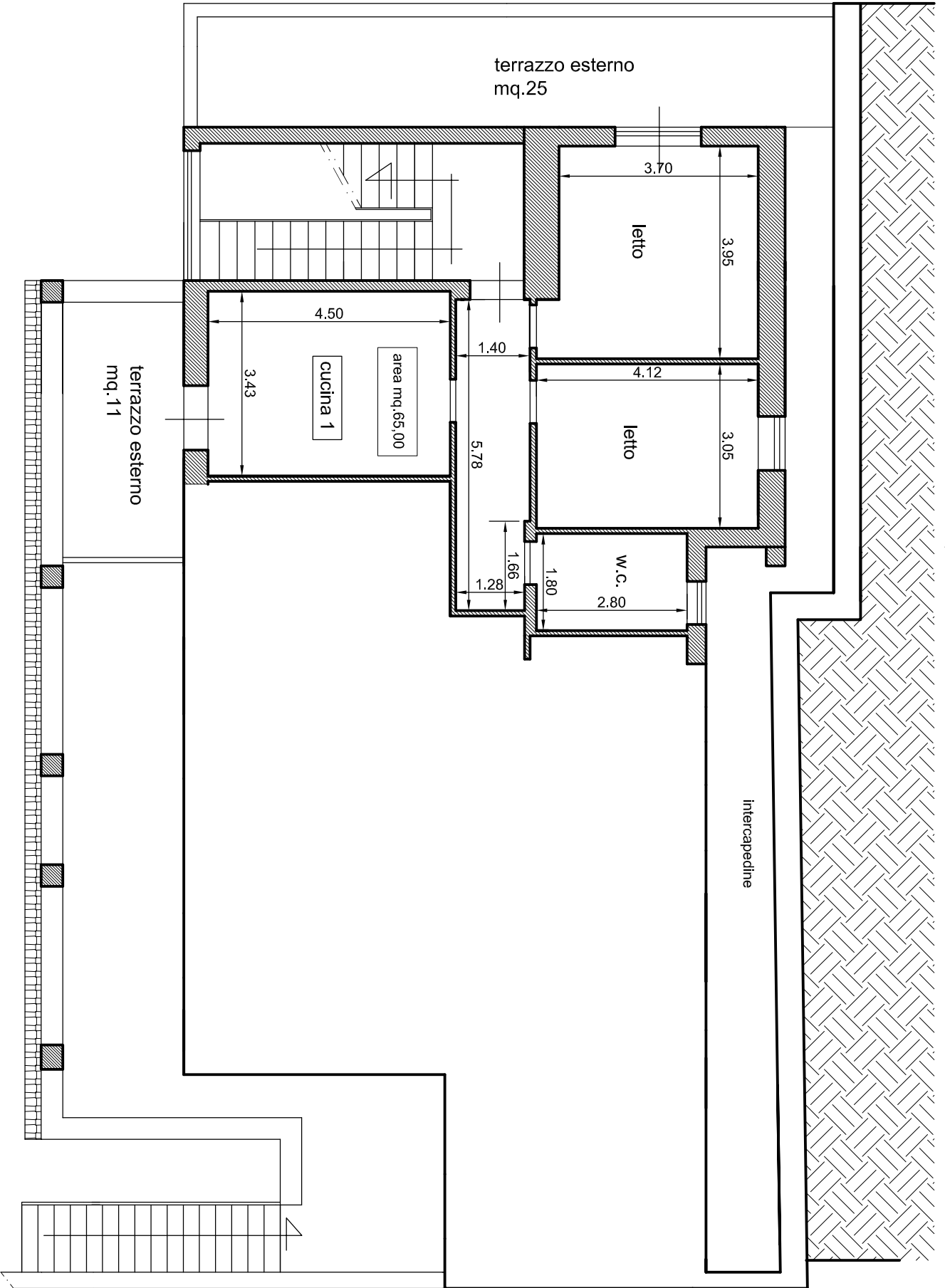
PIANTA PRIMO PIANO SOTTOSTRADA scala 1:100
